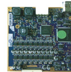
希望喷墨机通用喷头卡 HOPE PRINthead PROGRAM CARD
