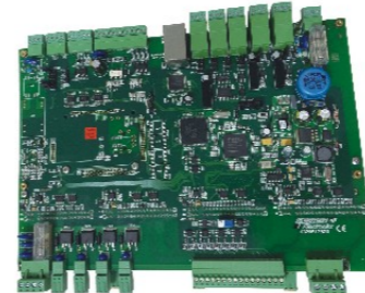
西施特姆喷头程序卡 SYSTEM PRINthead PROGRAM CARD
