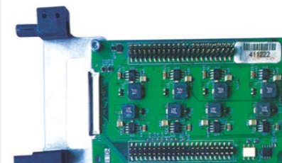
凯拉捷特喷头驱动卡 KERAJET DRIVE CARD
